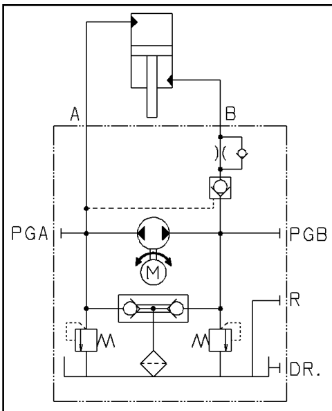
図1 油圧回路図
